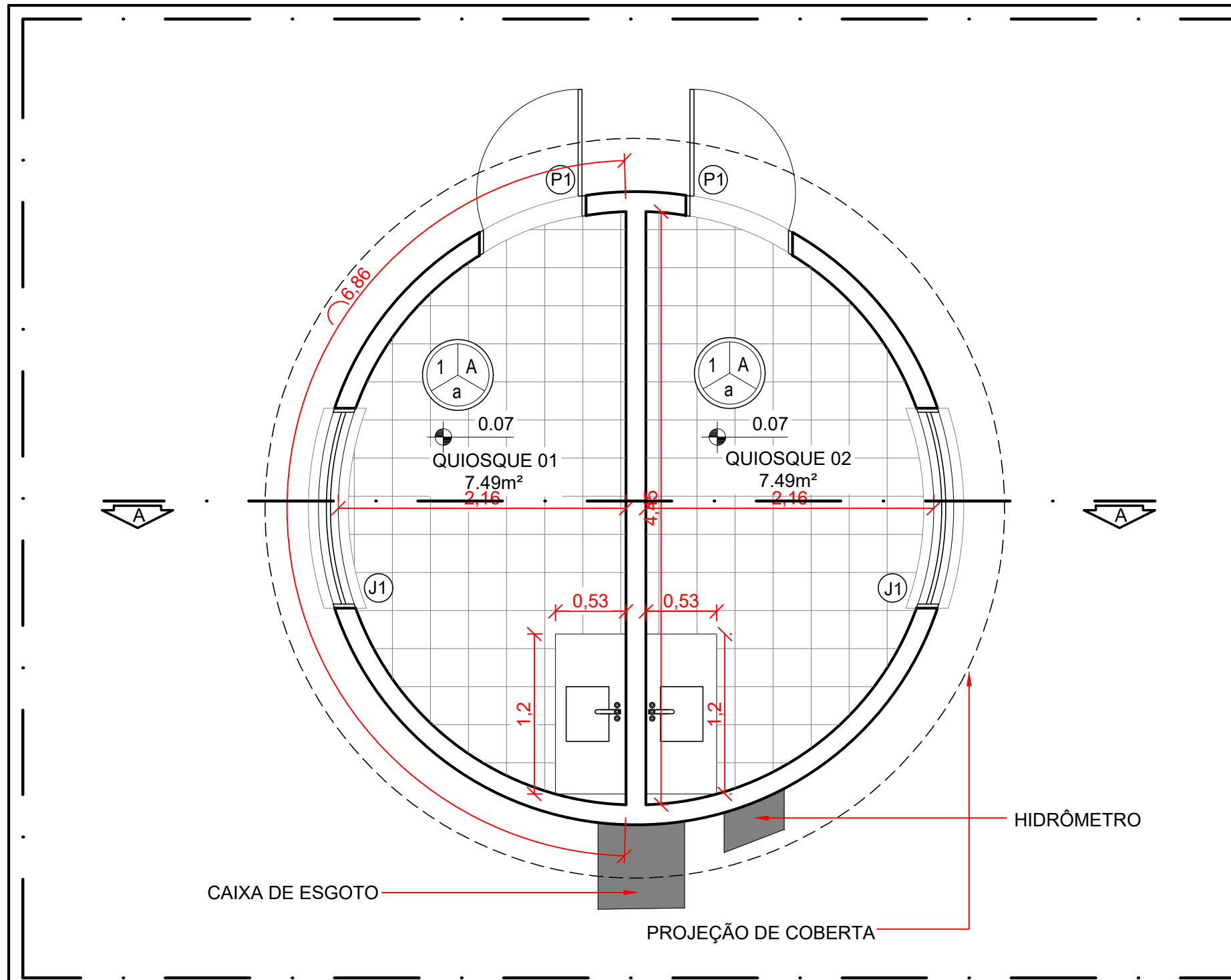
02 PLANTA BAIXA Escala 1/ 50
