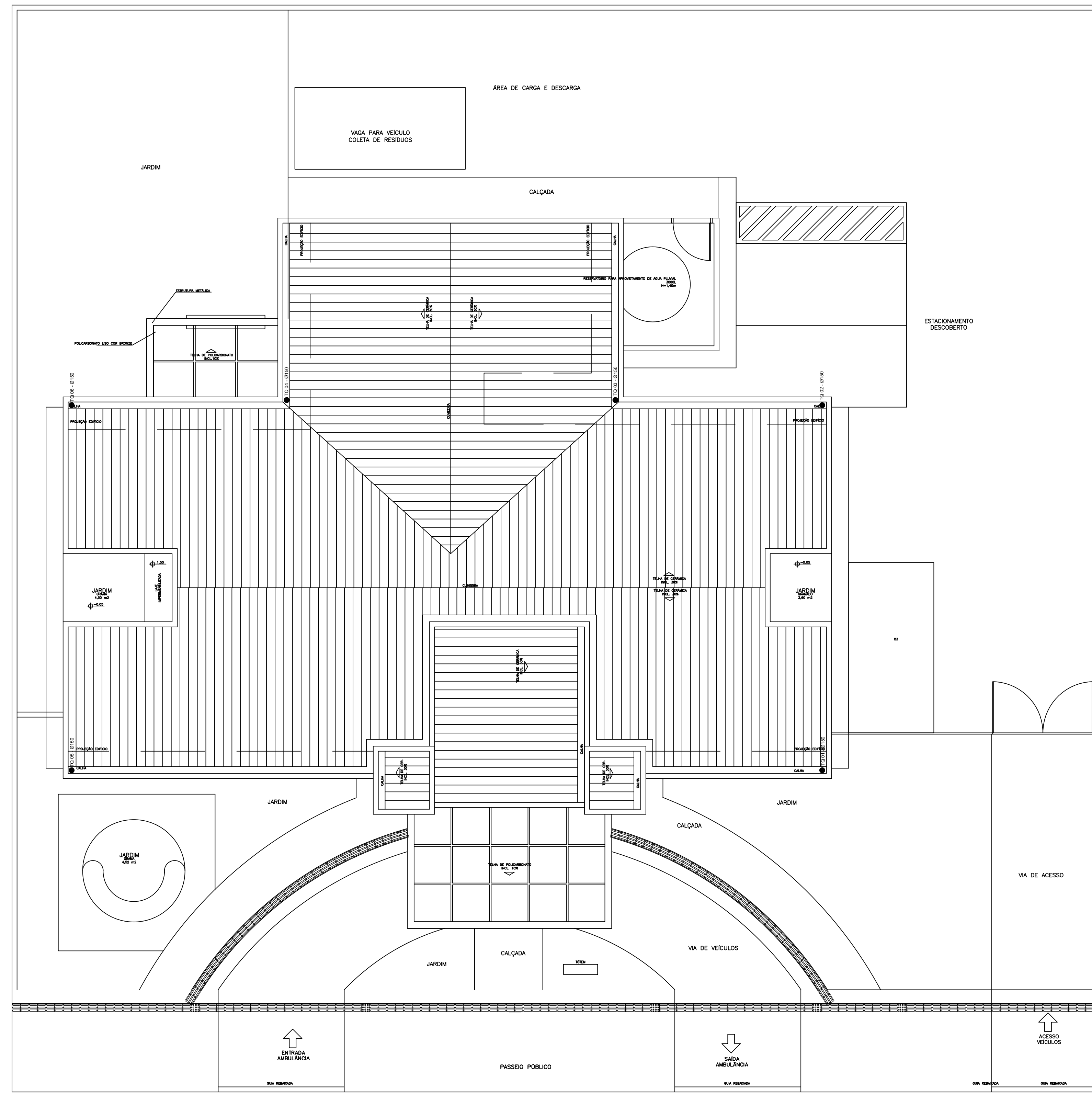
Planta Cobertura Escala: 1:50
