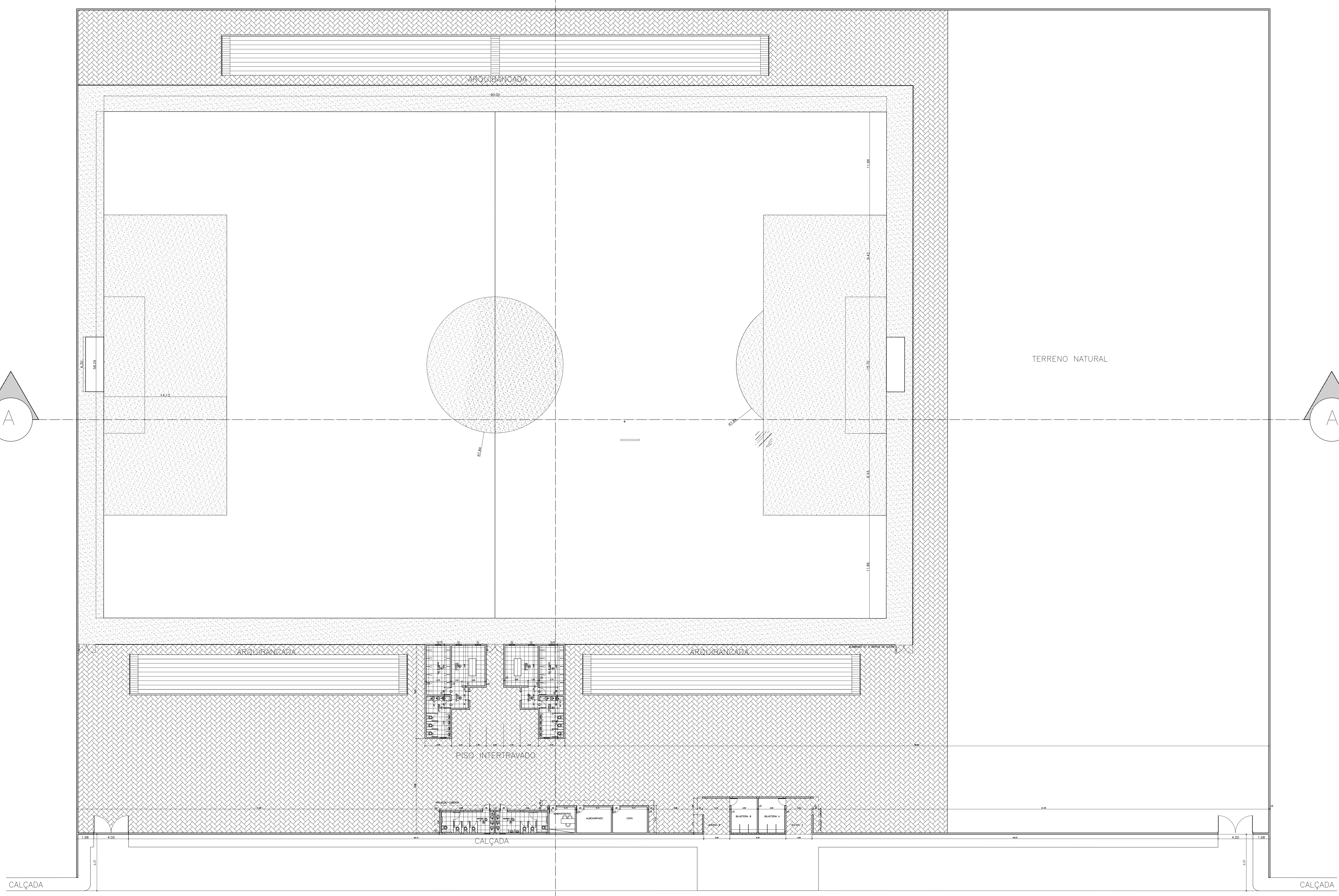
② PLANTA BAIXA ESTADIO DE FUTEBOL ESC. 1 250
